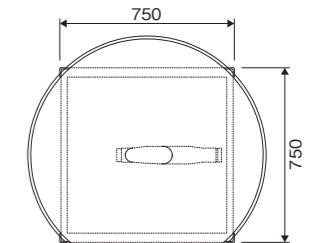
■OKH-1000MS寸法図
