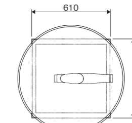
■OKH-800MS寸法図
